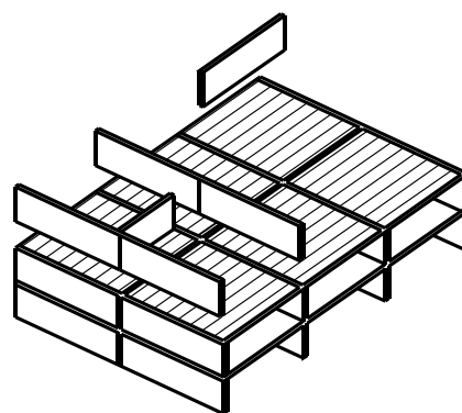
b) Structure constituée de refends ou d'éléments de voiles (structure formée de panneaux)
