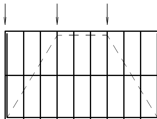
d) Plancher ou toiture formant diaphragme
