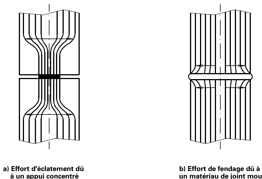
Figure 4.135 : Efforts transversaux dans les joints comprimés
