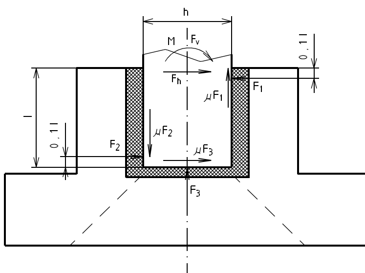
Figure 5.122 a) : Encuvement avec joint à parois nervurées
