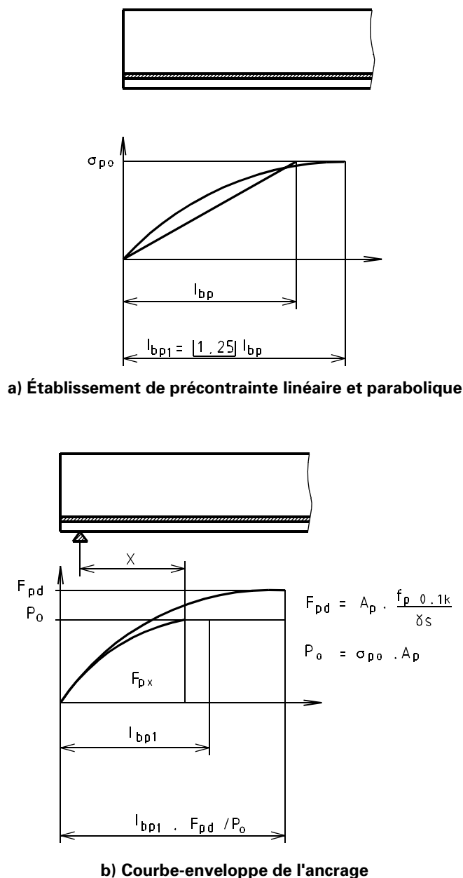
Figure 4.134 : Établissement de la précontrainte dans la zone de transfert
