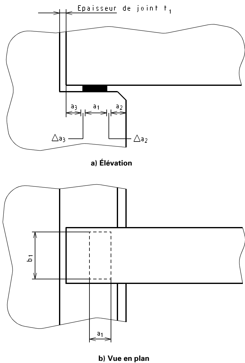
Figure 4.137 : Exemple de disposition d'appui
