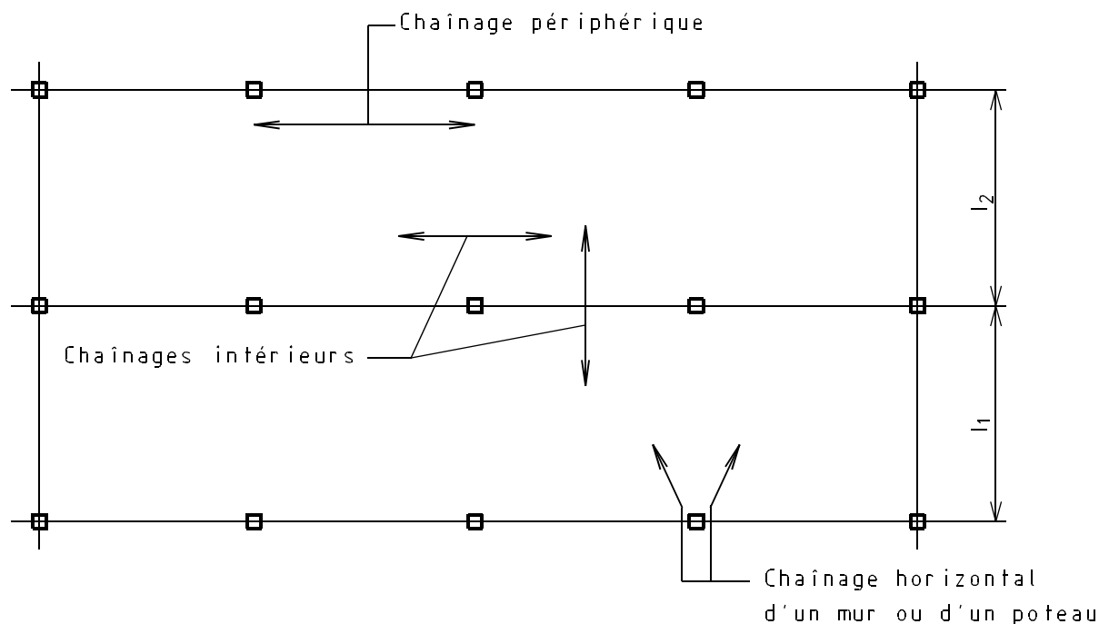
Figure 5.123 : Chaînages vis-à-vis des actions accidentelles
