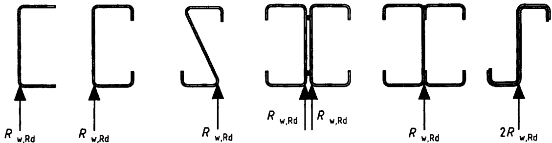
Figure 5.8 : Exemples de sections transversales ne comportant qu'une seule âme
