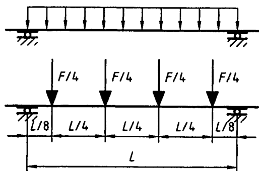
a) Chargement uniformément réparti et exemple d'une alternative avec charges linéaires équivalentes
