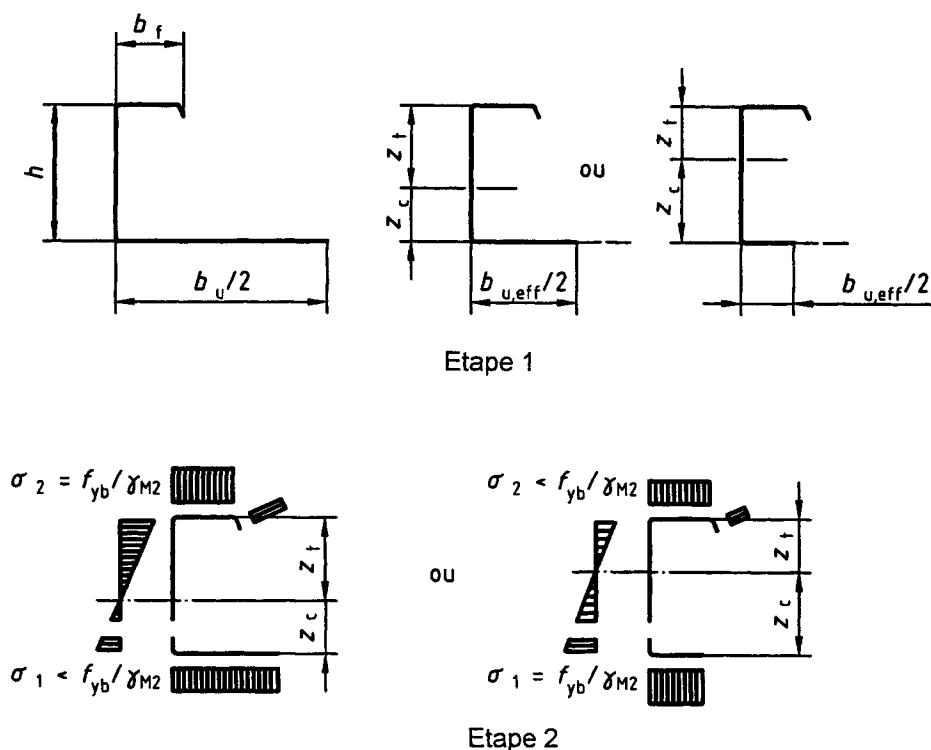
Figure 10.9 : Détermination du moment résistant - Plaque comprimée
