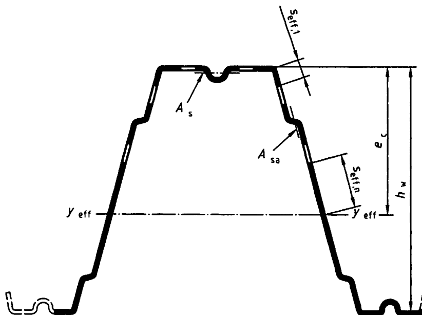
Figure 4.9 : Plaque nervurée munie de raidisseurs de plaque et de raidisseurs d'âme
