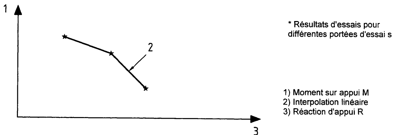
Figure A.8 : Interaction entre moment sur appui et réaction d'appui
