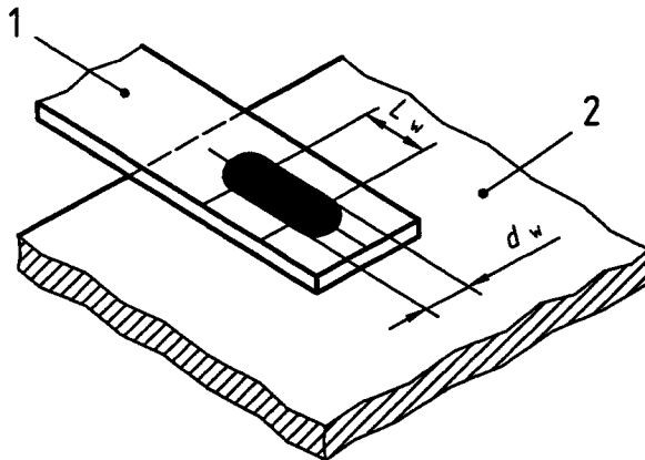
Figure 8.7 : Soudure oblongue par points à l'arc
