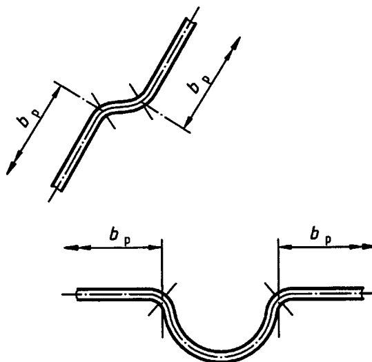
d) largeur de référence b_p de parois adjacentes à des raidisseurs
