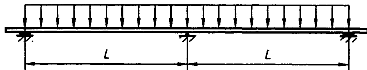
Figure A.3 : Montage d'essai pour essais en travée double
