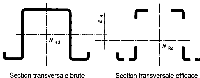
Figure 5.1 : Section transversale efficace en compression
