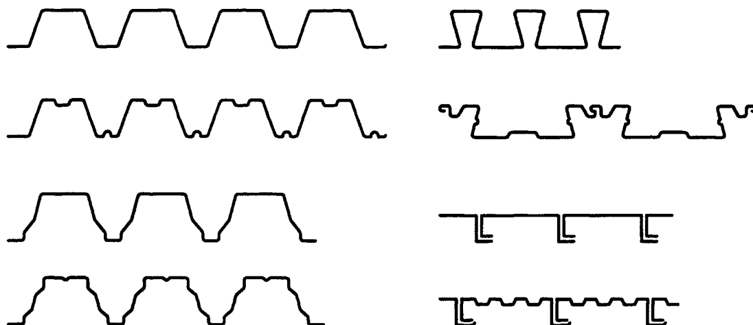
c) Plaques nervurées et plateaux
