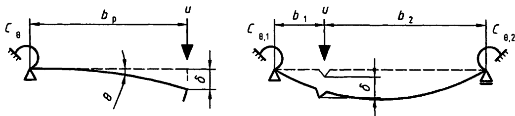
a) Système réel
