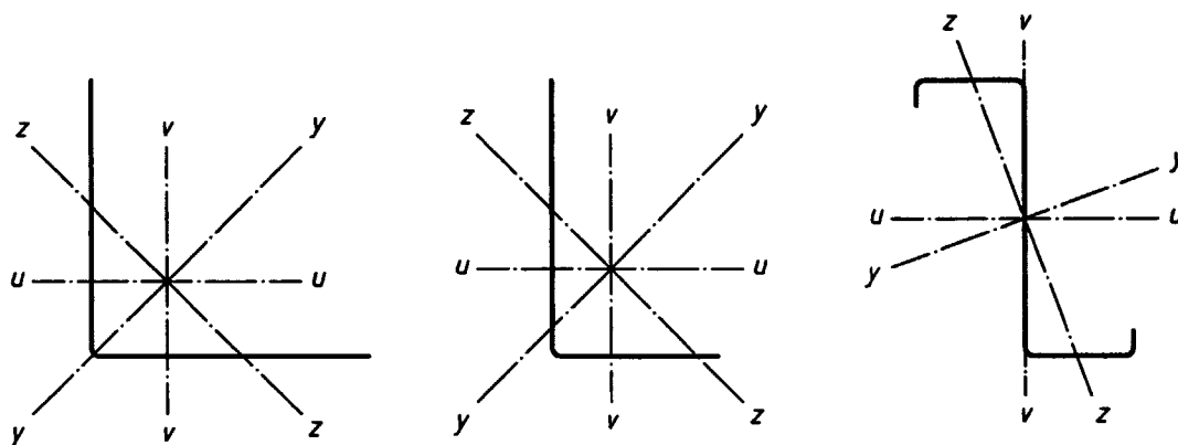
Figure 1.6 : Convention pour les axes
