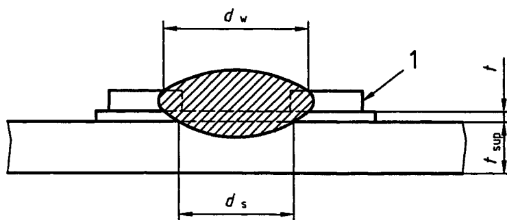
c) Une seule tôle assemblée avec rondelle pour soudure
