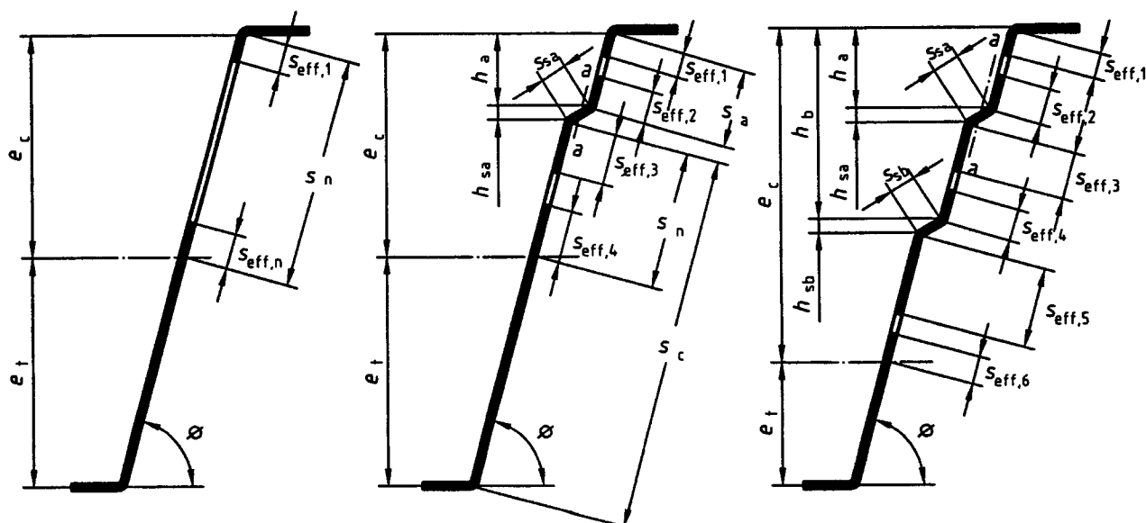
Figure 4.7 : Sections transversales efficaces d'âmes de plaques nervurées
