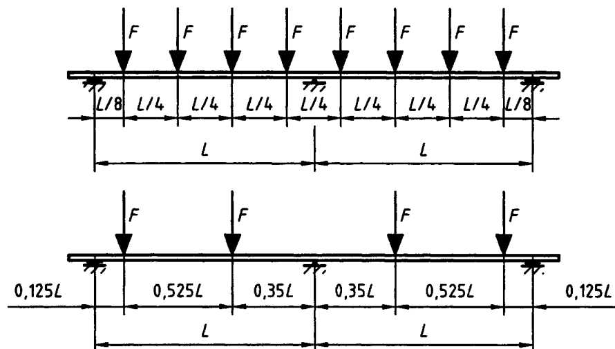
Figure A.4 : Exemples de dispositions appropriées de charges linéaires utilisées à titre d'alternative
