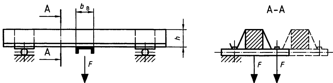
b) Appui intermédiaire soumis à un soulèvement simulé
