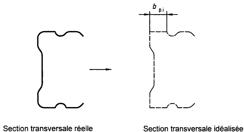
Figure 3.4 : Prise en compte approchée des angles arrondis
