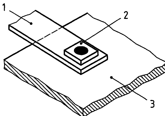
Figure 8.5 : Soudure par points à l'arc avec rondelle pour soudure
