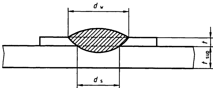
a) Une seule tôle assemblée ( \sum t = t )
