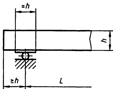
c) Exemple de dispositions d'appui destinées à empêcher la déformation de la section transversale
