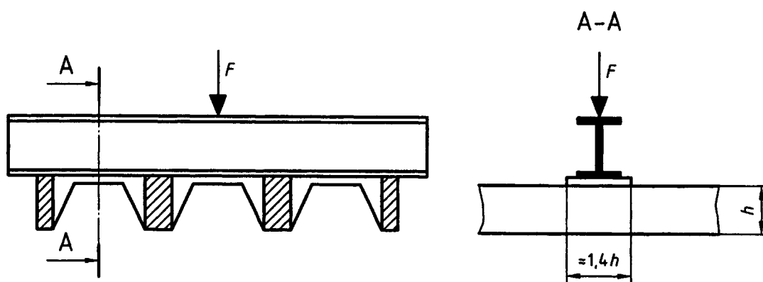
d) Exemple de méthode d'application d'une charge linéaire
