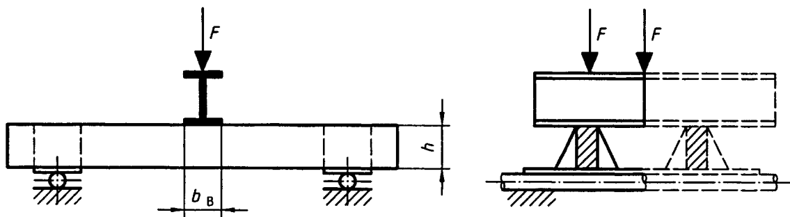
a) Appui intermédiaire soumis à un chargement de gravité
