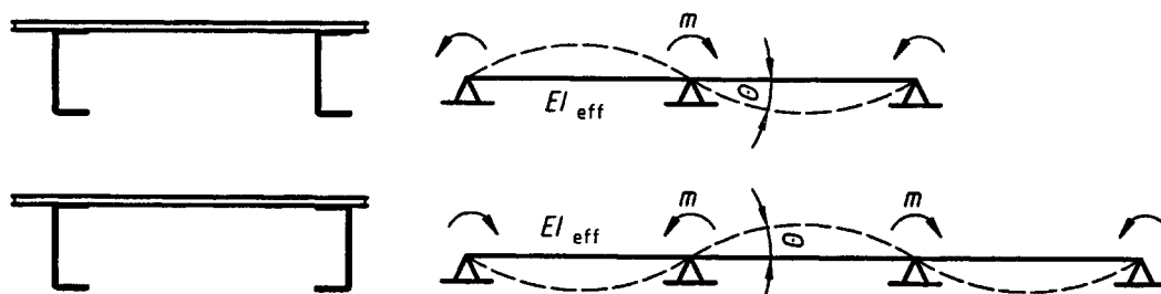
Figure 10.7 : Modèle pour le calcul de C_{D,C}
