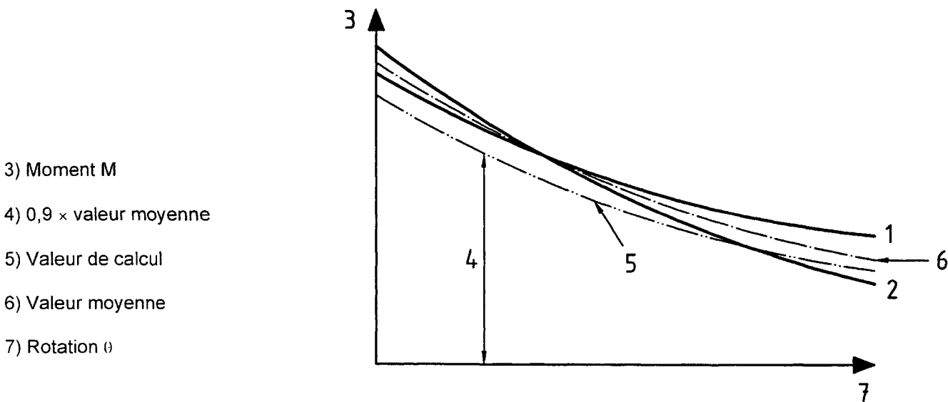
Figure A.10 : Déduction de la caractéristique moment-rotation de calcul
