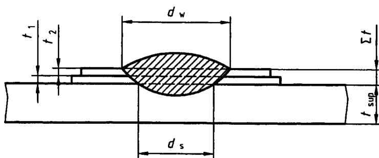
b) Deux tôles assemblées ( \sum t = t_1 + t_2 )
