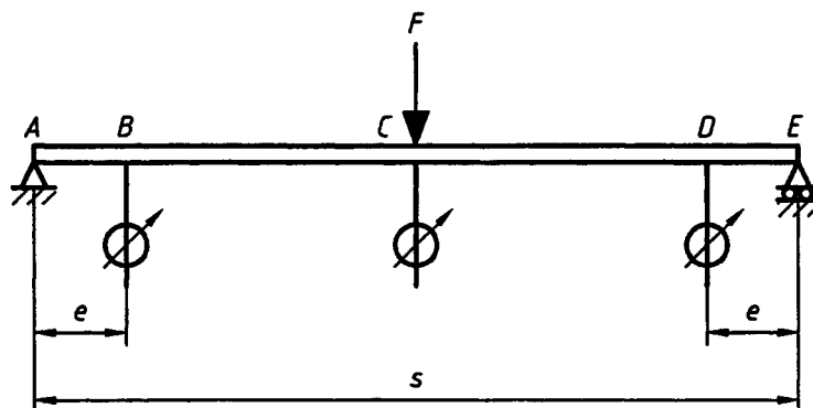
Figure A.7 : Dispositif pour essais d'appui intermédiaire
