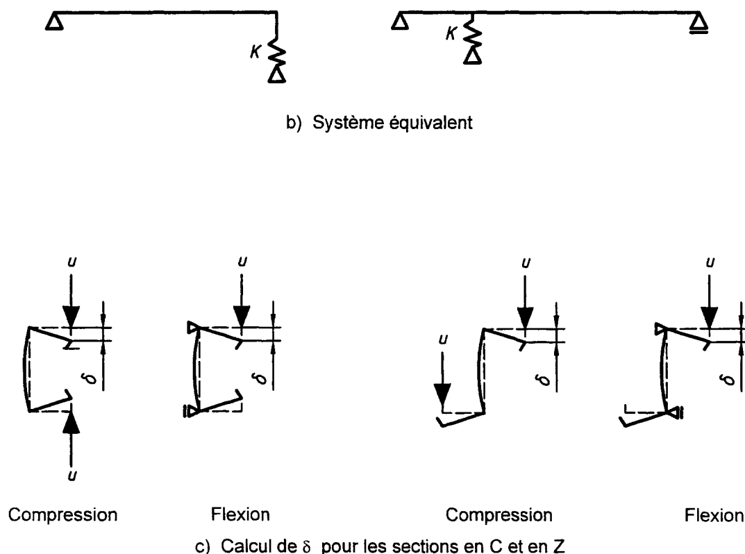
Figure 4.1 : Détermination de la rigidité du support élastique
