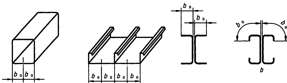
Figure 5.4 : Largeur b_0 contribuant au trainage de cisaillement
