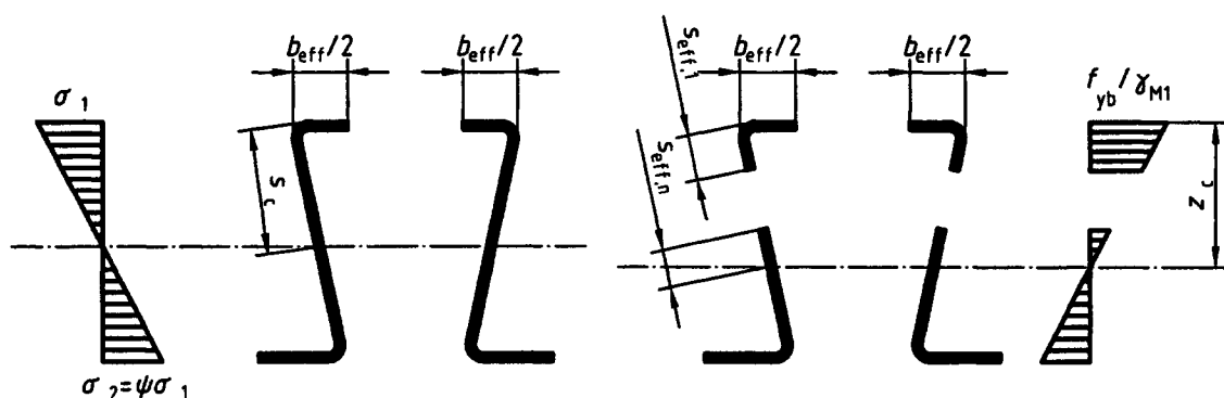
Figure 5.2 : Section transversale efficace pour la résistance aux moments fléchissants
