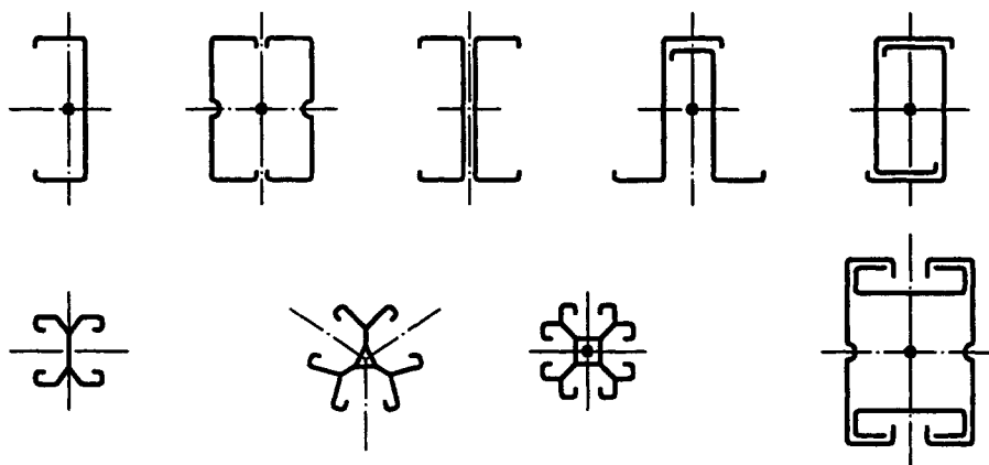
a) Barres comprimées et barres tendues
