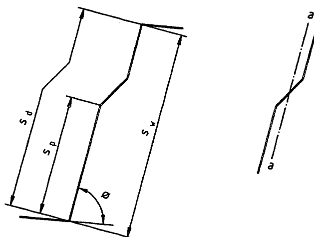
Figure 5.7 : Ame raidie longitudinalement
