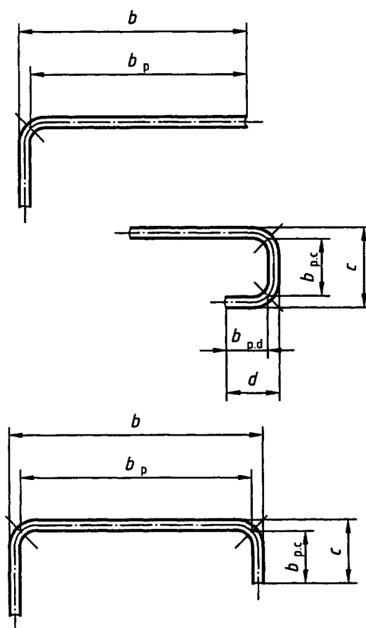
b) largeur de référence b_p des parois b, c et d
