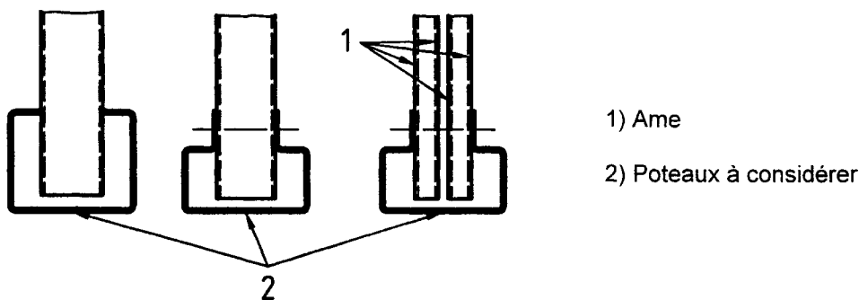
b) Assemblages capables d'assurer un maintien significatif à la torsion et au gauchissement
