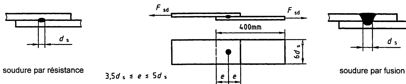
Figure 8.3 : Eprouvettes pour essais de cisaillement de soudures par points
