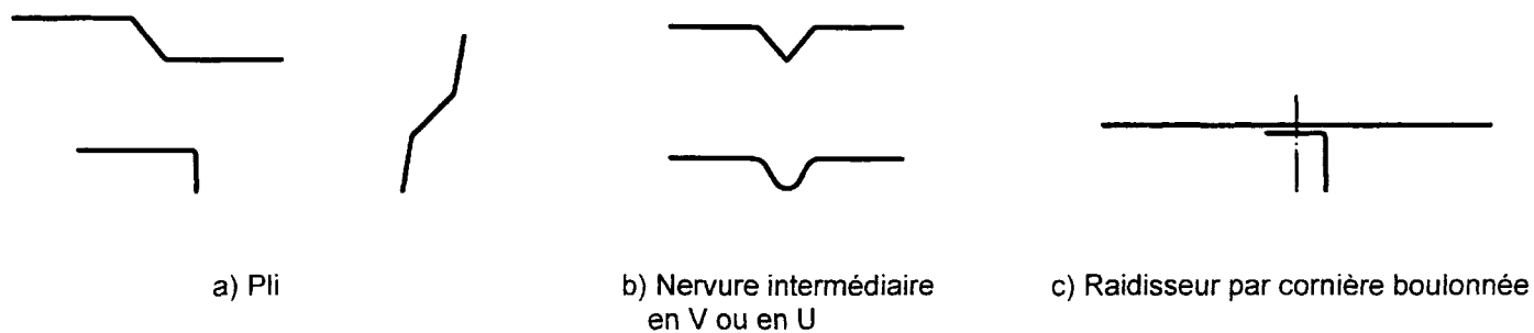
Figure 1.3 : Formes typiques de raidisseurs pour profilés et plaques formés à froid
