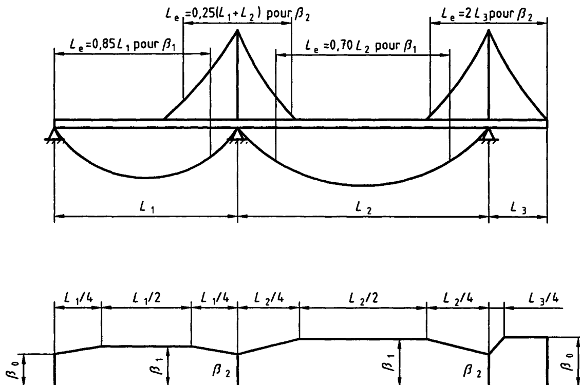
Figure 5.6 : Hypothèses simplifiées pour les poutres continues
