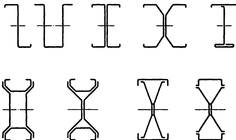
b) Poutres et autres barres fléchies
