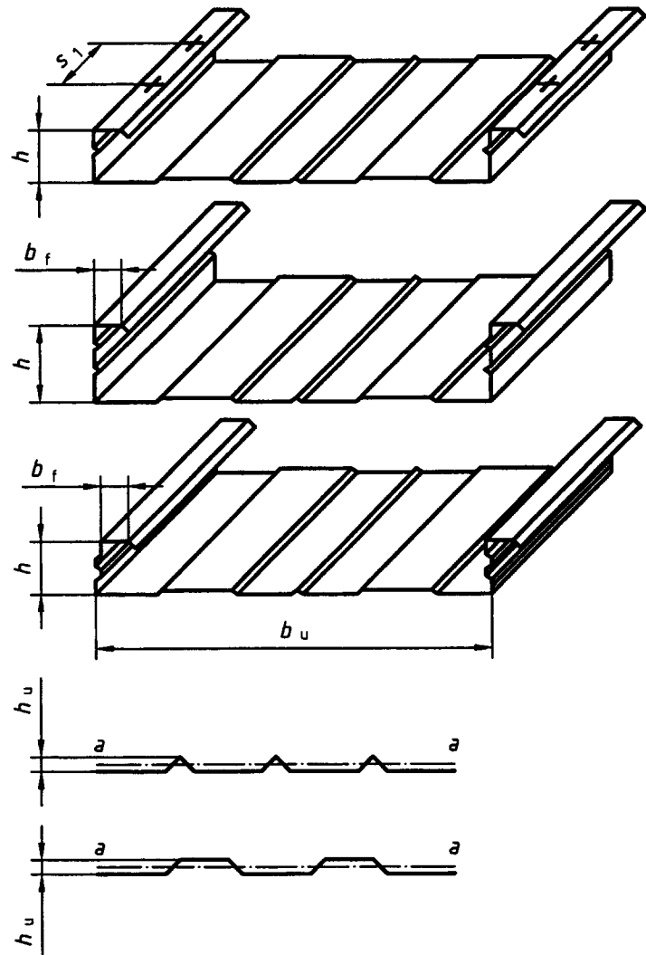
Figure 10.8 : Géométries typiques des plateaux
