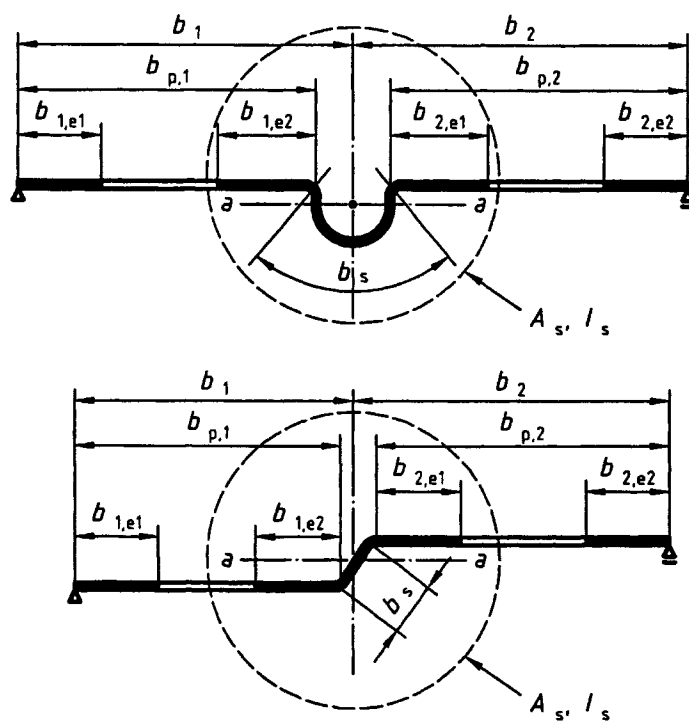
Figure 4.4 : Raidisseurs intermédiaires
