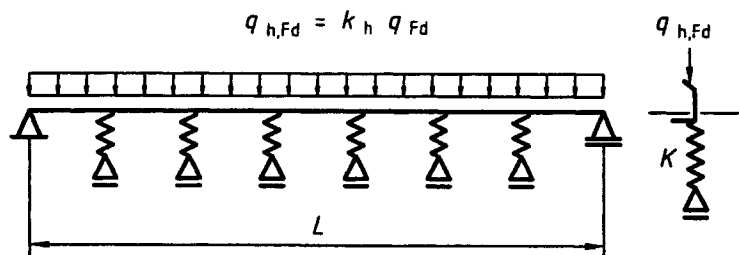
Figure 10.1 : Modélisation de pannes contreventées latéralement et maintenues en rotation par les plaques
