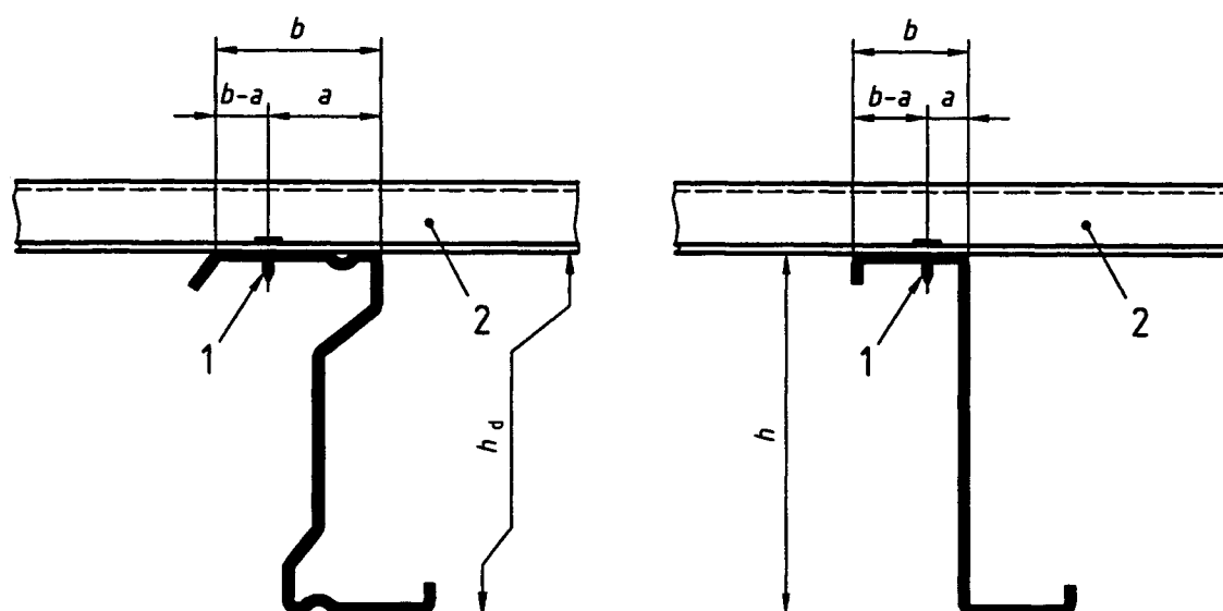
Figure 10.6 : Panne et plaques assemblées
