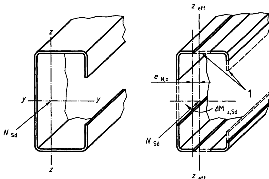
Figure 6.1 : Déplacement des axes centroïdes
