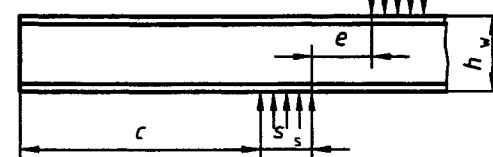
Figure 5.9 : Charges localisées et appuis - Sections transversales avec une seule âme
