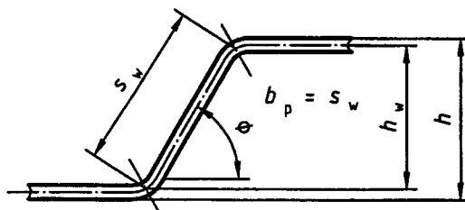
c) largeur de référence b_p pour une âme ( b_p = largeur inclinée s_w )
