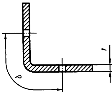
Figure 3.2 : Cornières comportant des trous dans les deux ailes
