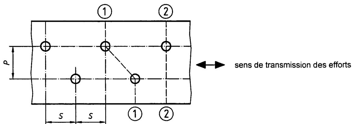
Figure 3.1 : Trous en quinconce et sections s'y rapportant
