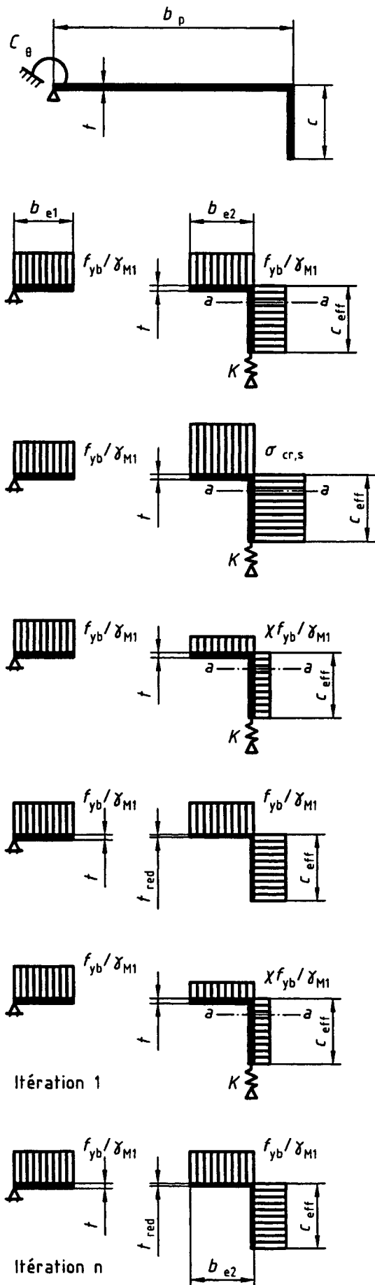
Figure 4.3 : Résistance à la compression d'une semelle munie d'un raidisseur de bord
