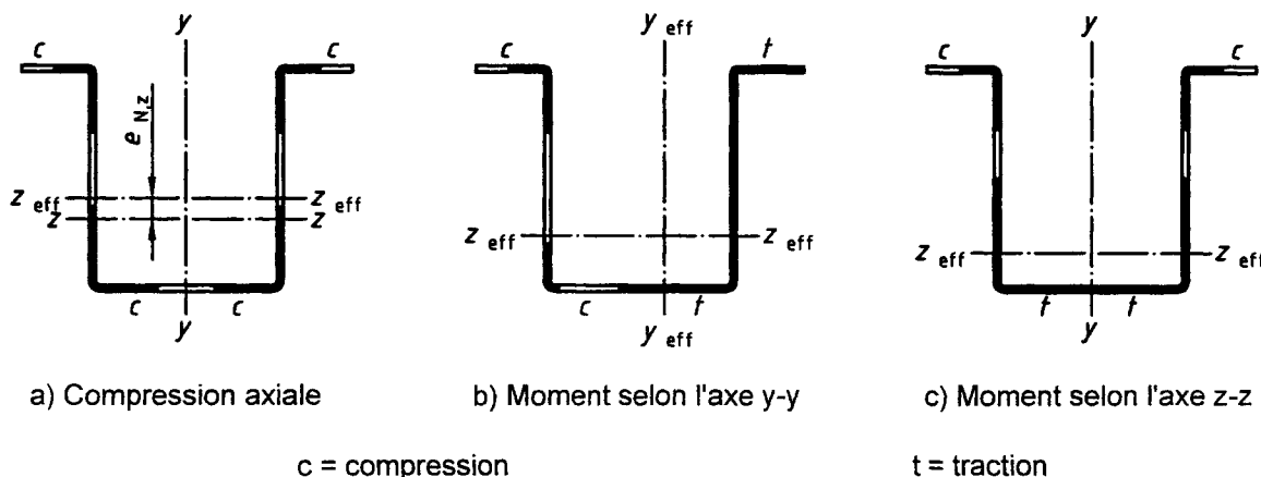
Figure 6.6 : Calcul des caractéristiques de section efficace
