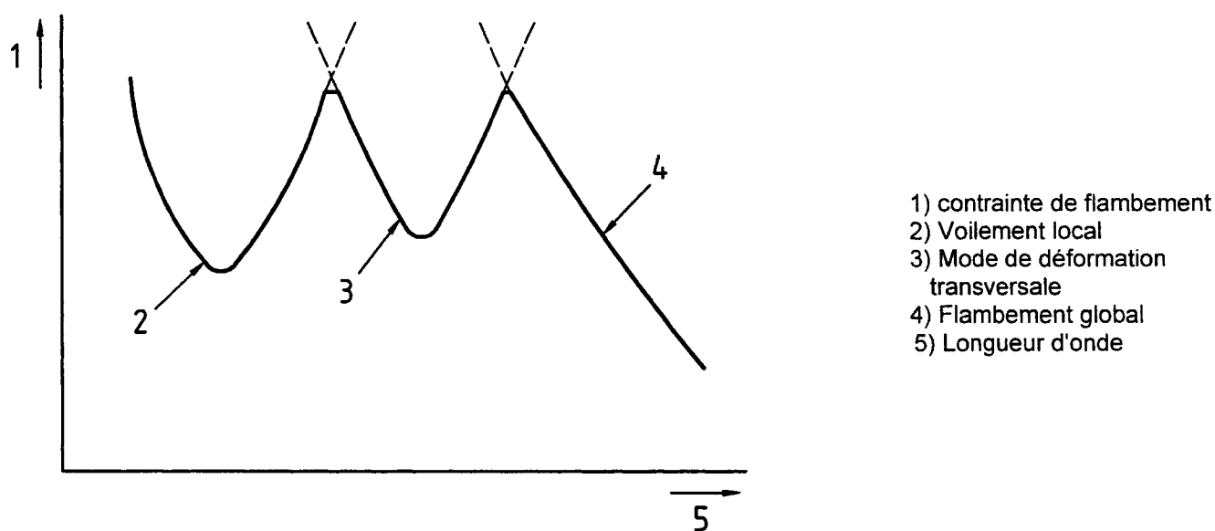
Figure 6.5 : Contraintes critiques élastiques pour divers modes de ruine
