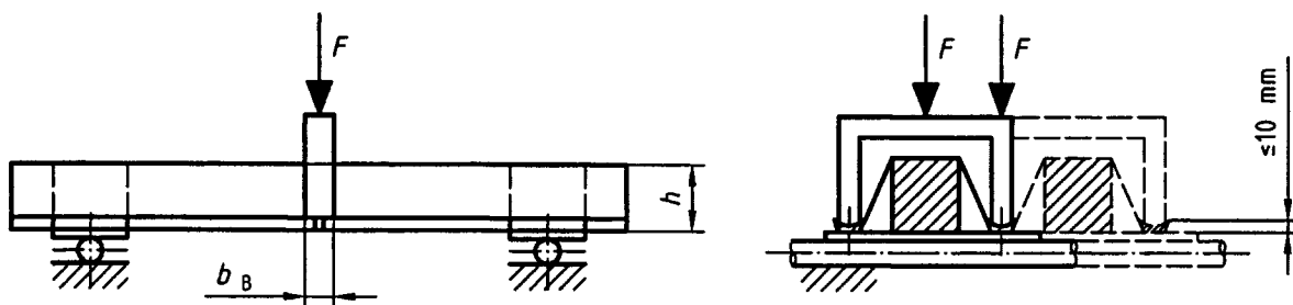
c) Appui intermédiaire supportant un chargement appliqué sur la semelle tendue
