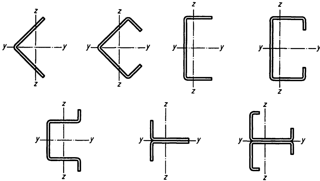
Figure 6.2 : Sections transversales sujettes au flambement par flexion-torsion
