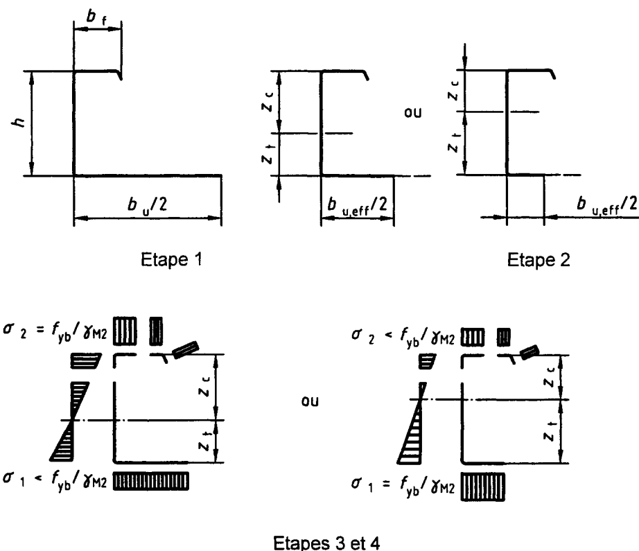
Figure 10.10 : Détermination du moment résistant - Plaque tendue
