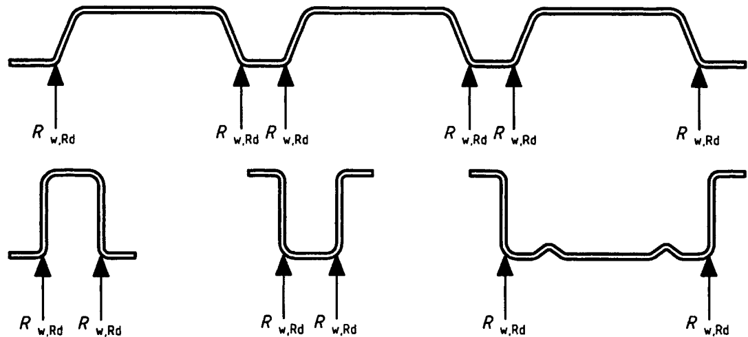
Figure 5.10 : Exemples de sections transversales comportant deux âmes ou plus
