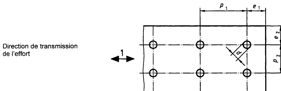
Figure 8.1 : Pince longitudinale, pince transversale et espacement des fixations et des soudures par points
