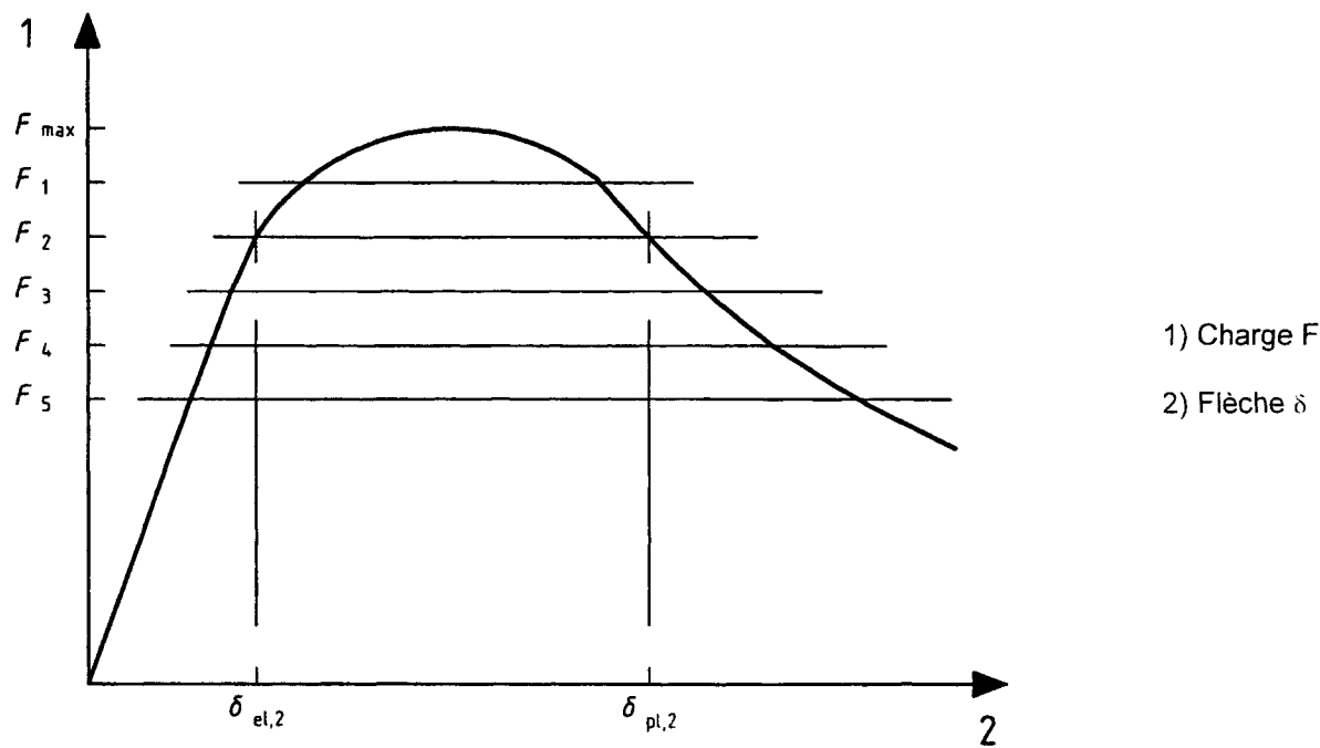
Figure A.9 : Relation entre charge et flèche nette
