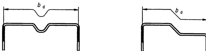
Figure 5.5 : Largeur développée b_d de semelles munies de raidisseurs intermédiaires
