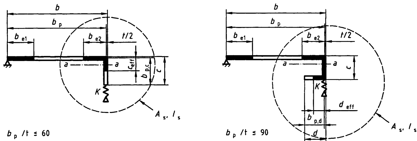
Figure 4.2 : Raidisseurs de bord
