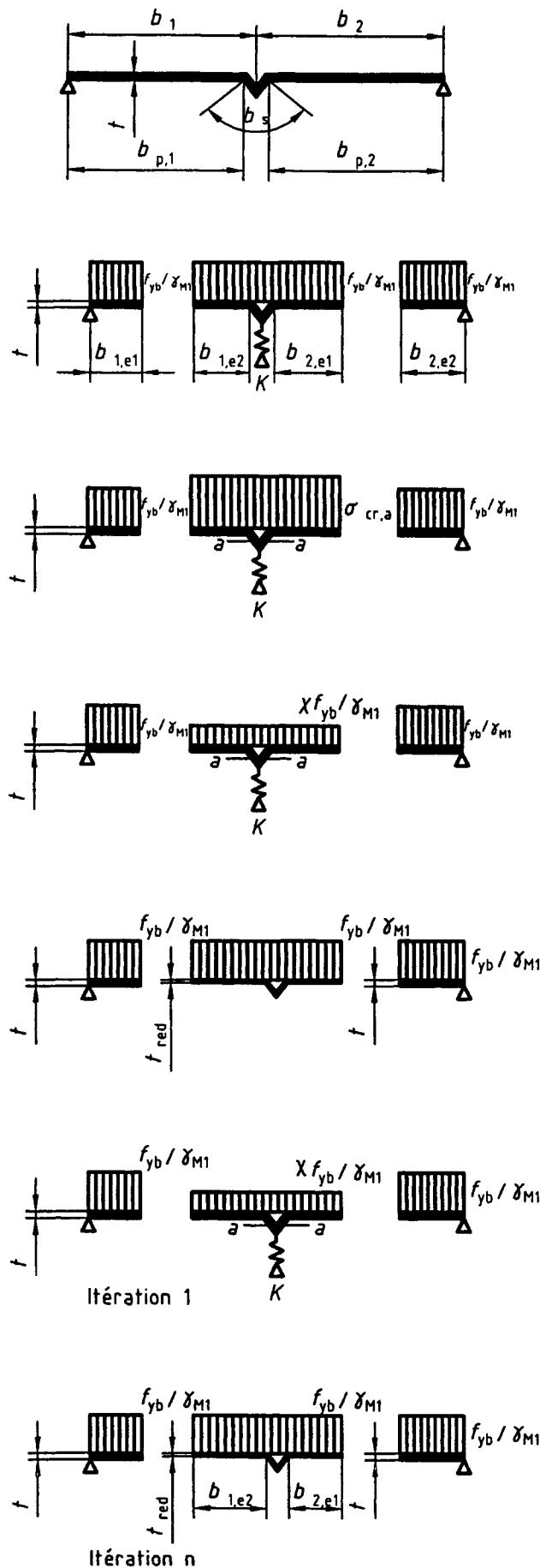
Figure 4.5 : Résistance à la compression d'une semelle munie d'un raidisseur intermédiaire
