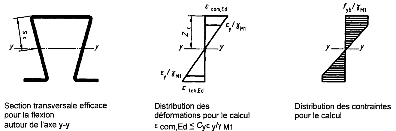
Figure 5.3 : Moment résistant partiellement plastique
