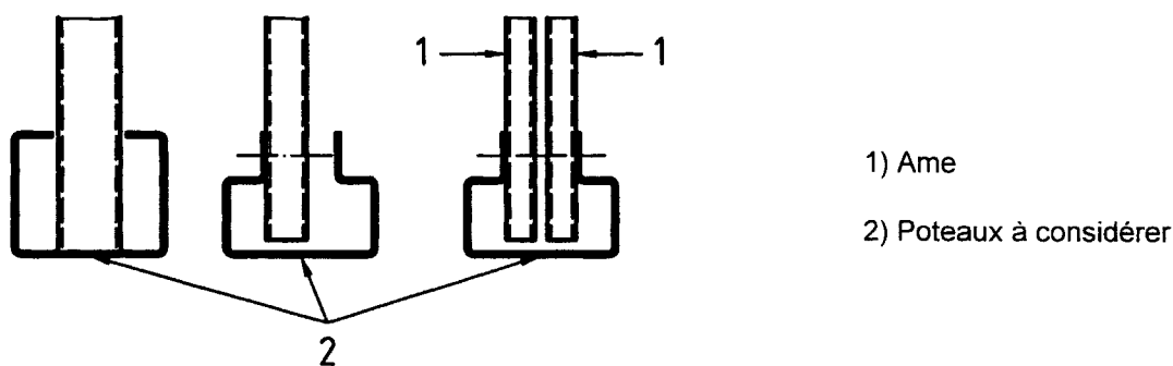
a) Assemblages capables d'assurer un maintien partiel à la torsion et au gauchissement
