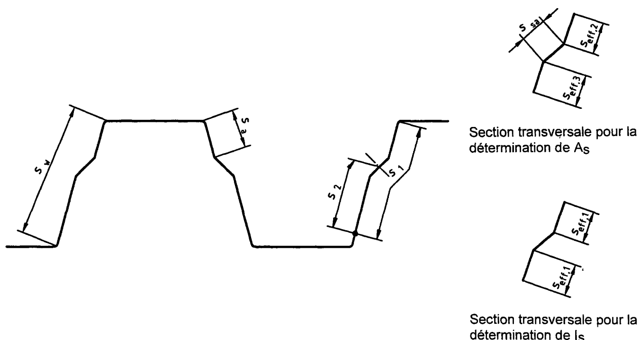
Figure 4.8 : Raidisseurs d'âmes de plaques nervurées
